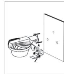
Τοποθέτηση σε τοίχο Wall Mounting
